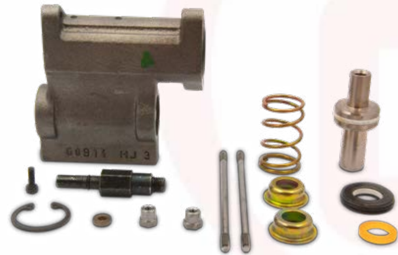
9577831 CONJUNTO ACIONAMENTO PNEUMÁTICO TC57 TC59 FLUTUAÇÃO APLICAÇÃO + TC5070 / TC5090
