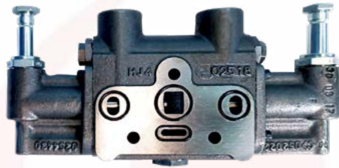
DQ44174 CORPO COMANDO ELÉTRICO COLHEITADEIRA CONTROLE POSIÇÃO
