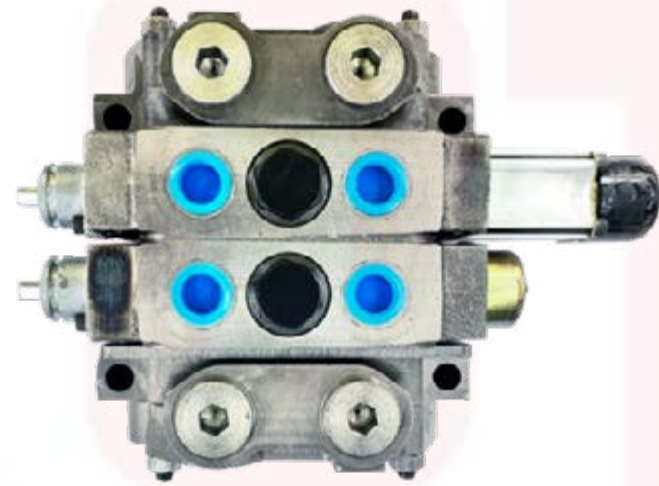
87346450 - COMANDO HIDRÁULICO V10 - APLICAÇÃO TM 110/TM140/TM150/7040
